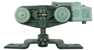
Laufwagen mit Aufhängewinkel – 1 Paar je Flügel –
