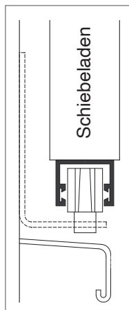
Winkel und Gleiter
