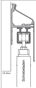
Schiebeläden „standard“ Profilkit mit Blende
