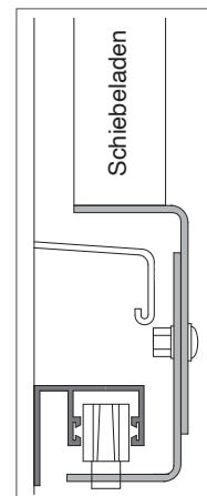
Schiene mit L-Lappen und verstellbare U-Winkel
