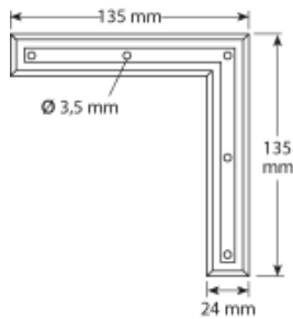
Ladenwinkel
