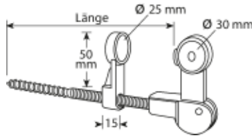
Standard-Ladenfeststeller
