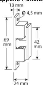
Kugelschnapper für gekuppelte Fensterläden
