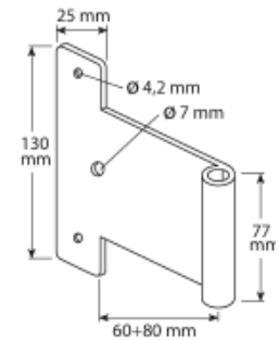
Standard-Ladenscharnier gekröpft (bei gekuppelten Läden)
