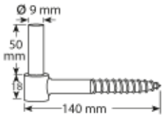
Standard-Schraubkloben
