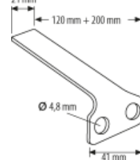
Riegelanschlag zu Ladenriegel (Schema 4 – über die Leibung)
