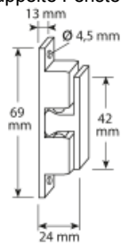
Kugelschnapper für gekuppelte Fensterläden
