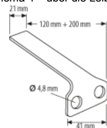
Riegelanschlag zu Ladenriegel (Schema 4 – über die Leibung)
