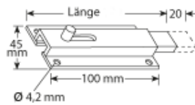
Ladenriegel (Länge 120+220 mm)
