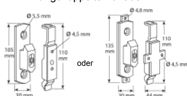
Ladenhalter für gekuppelte Türkläden
