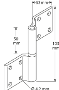
Standard-Ladenscharnier gekröpft (bei gekuppelten Läden)
