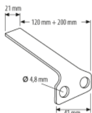
Riegelanschlag zu Ladenriegel
