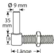
Schraubkloben M10 Innengewinde zu Isoblock oder Trägerplatte
