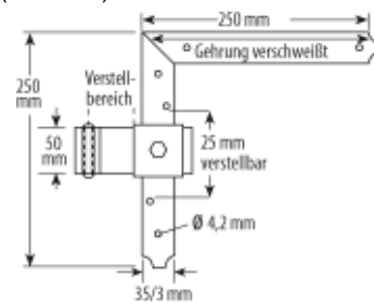
Schnellmontage-Winkelband vertikal und horizontal verstellbar (alternativ)
