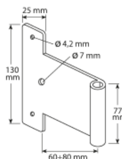
Winkelmittelband (Mitte Türflügel)
