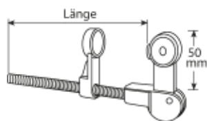
Ladenfeststeller M10 Innengewinde zu Isoblock oder Trägerplatte
