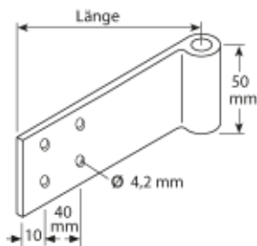
Standard-Ladenband
