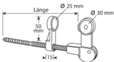
Standard-Ladenfeststeller
