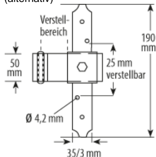
Schnellmontage-Kreuzband vertikal und horizontal verstellbar (alternativ)
