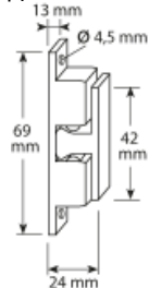
Kugelschnapper für gekuppelte Fensterläden
