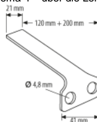
Riegelanschlag zu Ladenriegel (Schema 4 – über die Leibung)
