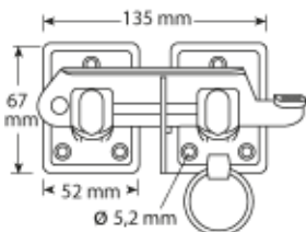
Standard-Ladenverschluss
