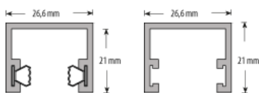
Führungsschiene unten (mit / ohne Gleitkeder)
