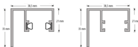
Führungsschiene unten mit L-Lappen (mit / ohne Gleitkeder)
