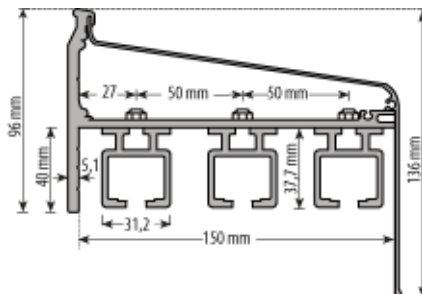
Profilkit Schiebeladen 3-spurig
