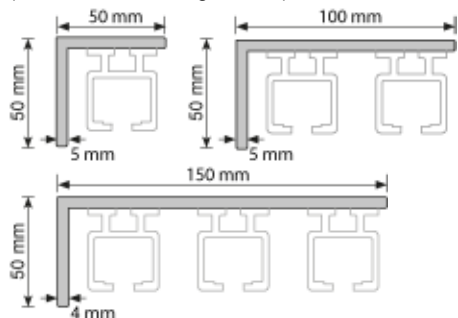
Alu-Winkel 1-spurig, 2-spurig, 3-spurig (ohne obere Führungsschiene)
