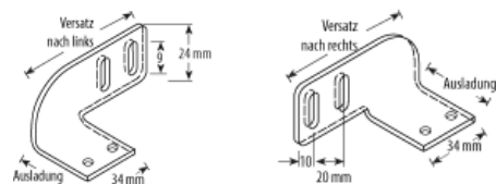
Versetzter Befestigungswinkel
