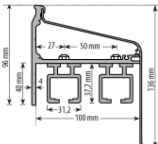
Profilkit Schiebeladen 2-spurig
