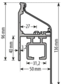
Profilkit Schiebeladen 1-spurig
