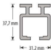
Obere Führungsschiene (einzeln)
