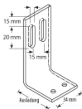
Befestigungswinkel
