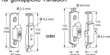
Ladenhalter für gekoppelte Türläden
