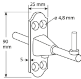
Kegel schmal*
