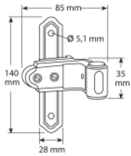
Ladenkreuzband
