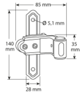
Ladenkreuzband
