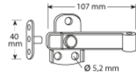
Einflügelladenverschluss
